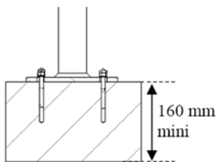
Fixation sur béton
