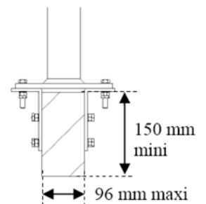
Fixation sur poutre lamellée collée
